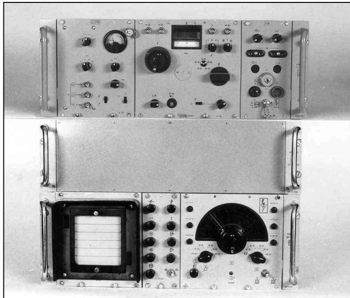
A VU-21M vevő és az UP-3MA panoráma
